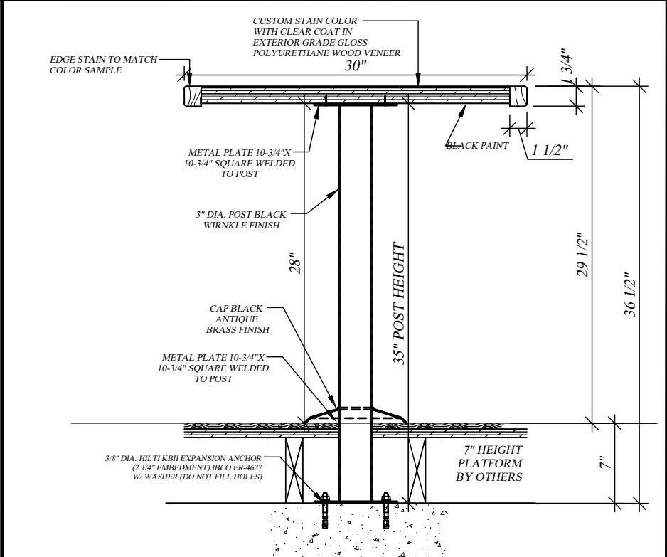
Q SECTION SCALE: 1"=1'-00"
