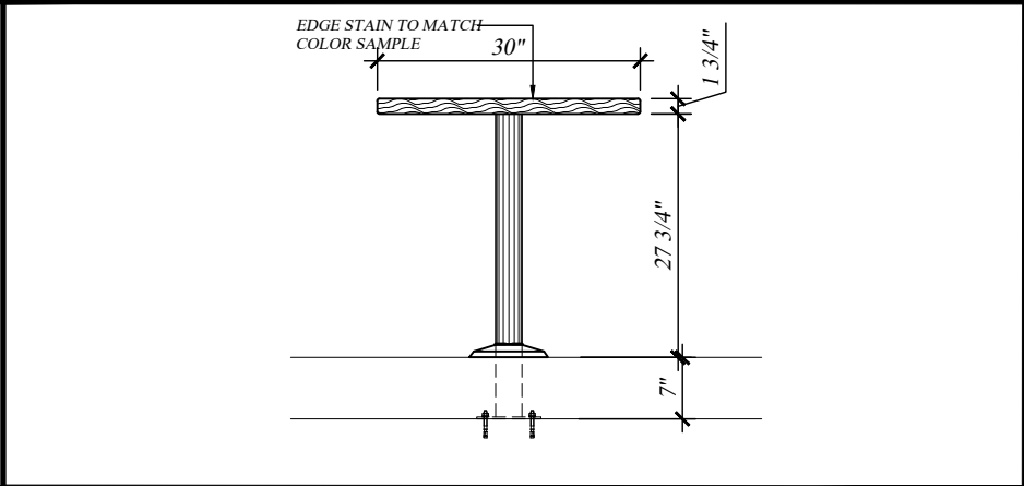
15 ELEVATION SCALE: 1/2"=1'-00"
