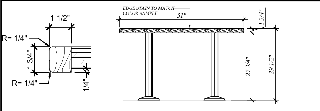
10 ELEVATION SCALE: 1/2"=1'-00"
