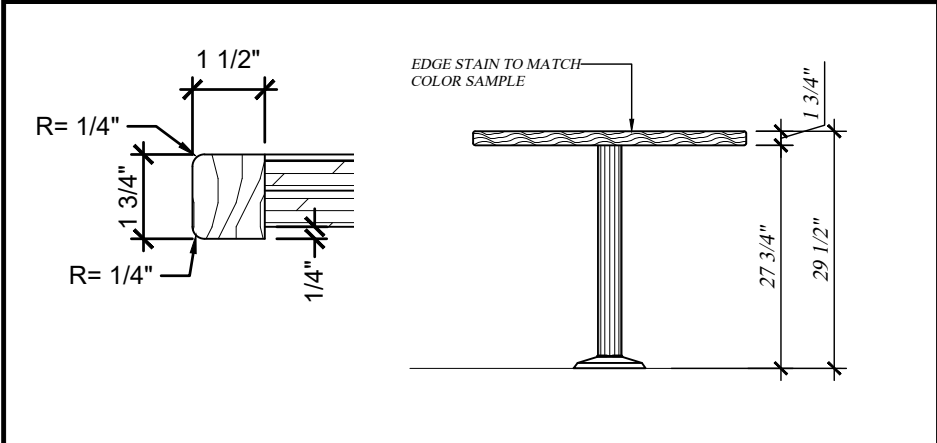
4 ELEVATION SCALE: 1/2"=1'-00"
