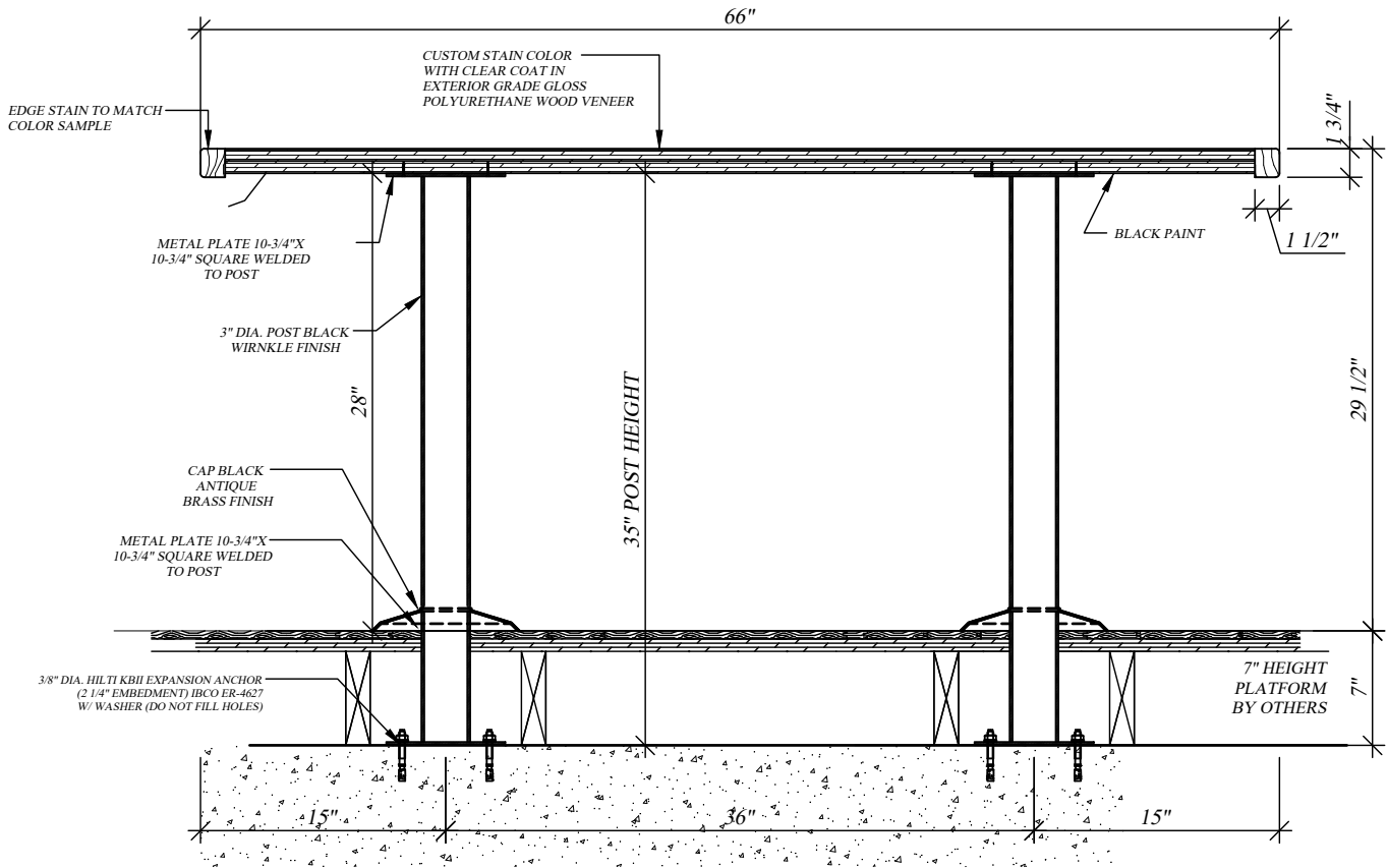
R ELEVATION SCALE: 1/2"=1'-00"
