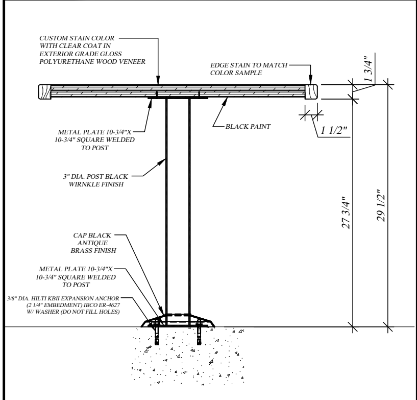
G SECTION SCALE: 1"=1'-00"
