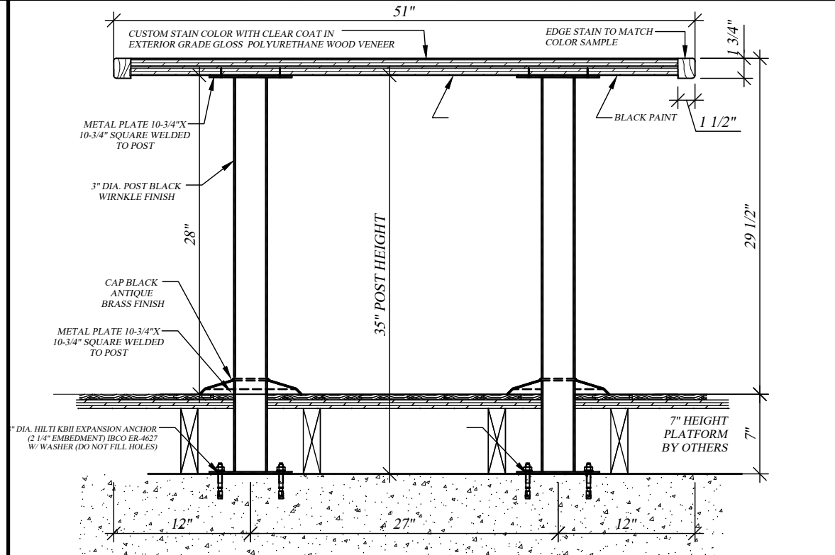
J SECTION SCALE: 1"=1'-00"
