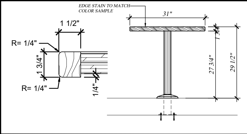
8 ELEVATION SCALE: 1/2"=1'-00"
