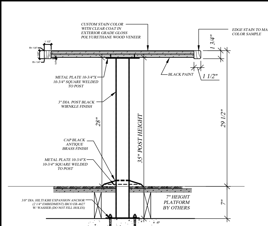
E SECTION SCALE: 1"=1'-00"
