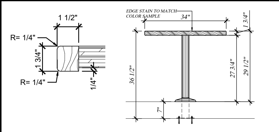
5 ELEVATION SCALE: 1/2"=1'-00"
