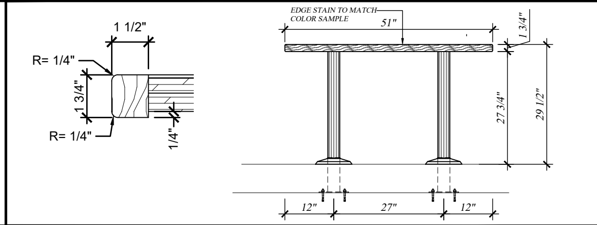
9 ELEVATION SCALE: 1/2"=1'-00"
