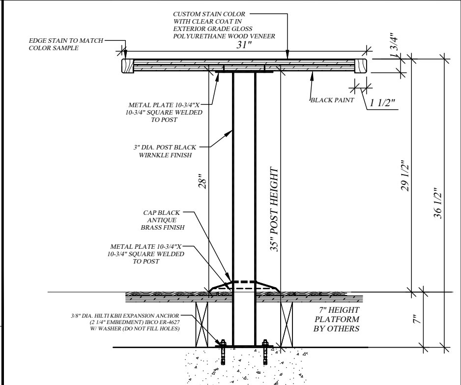
P SECTION SCALE: 1"=1'-00"
