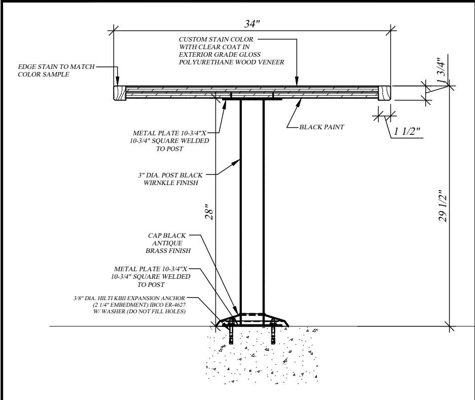
D SECTION SCALE: 1"=1'-00"
