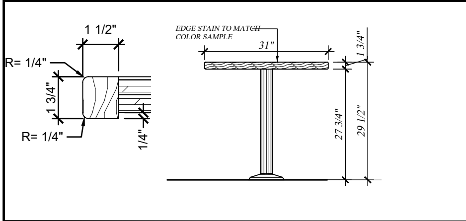
13 ELEVATION SCALE: 1/2"=1'-00"
