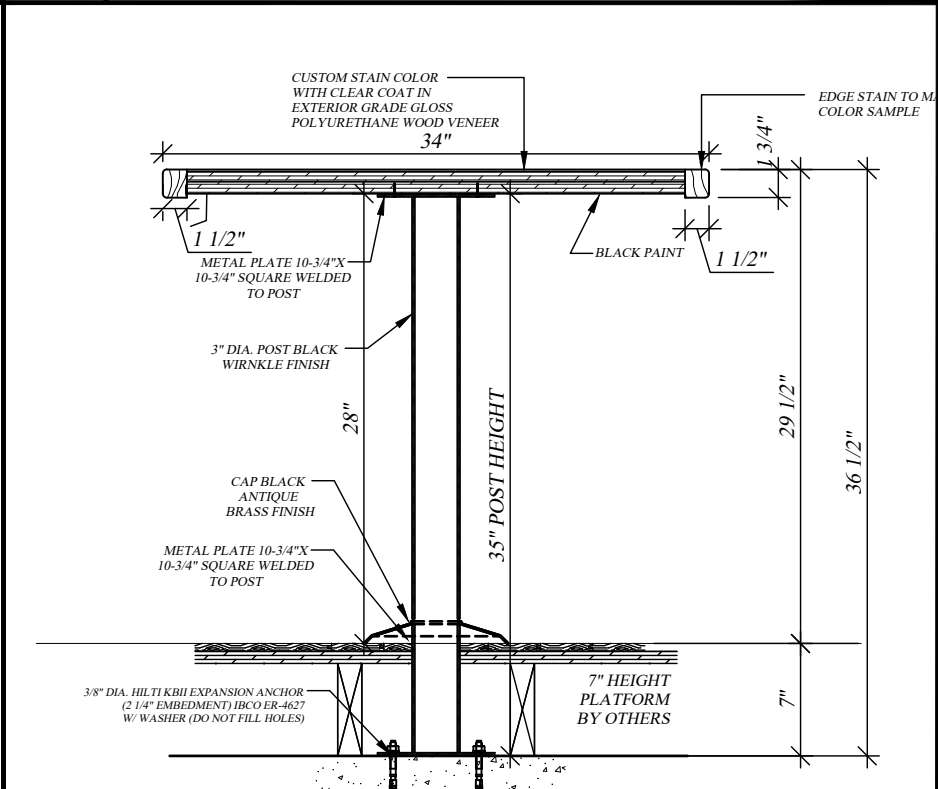
F SECTION SCALE: 1"=1'-00"
