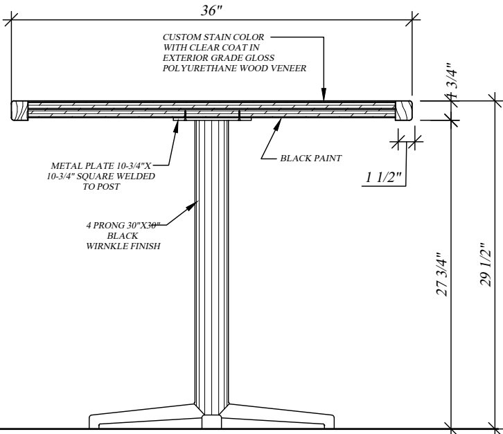
T ELEVATION SCALE: 1/2"=1'-00"
