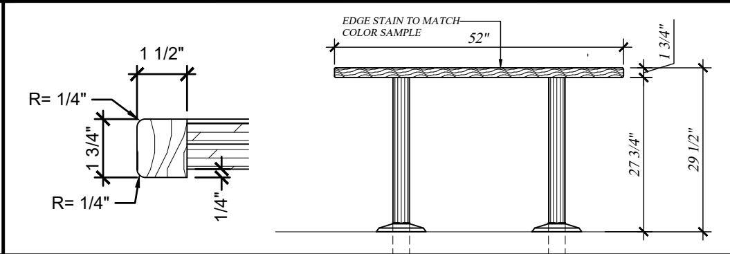
11 ELEVATION SCALE: 1/2"=1'-00"
